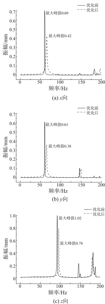
图 7 优化后整机三个方向上幅值与激振频率曲线
