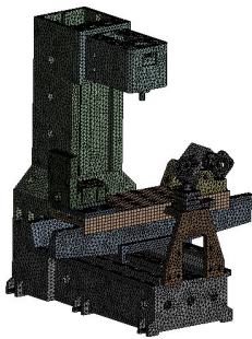
图3 有限元模型
