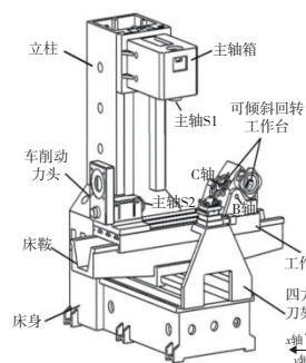
图1 多功能复合机床简化模型
